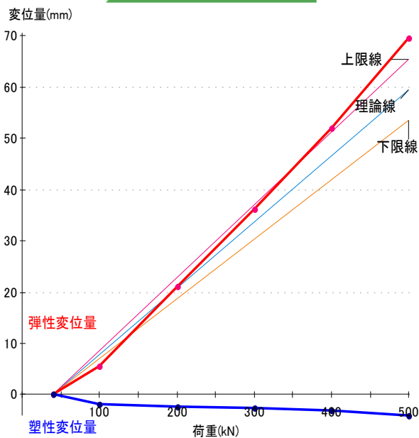
荷重-塑性・弾性変位量曲線
