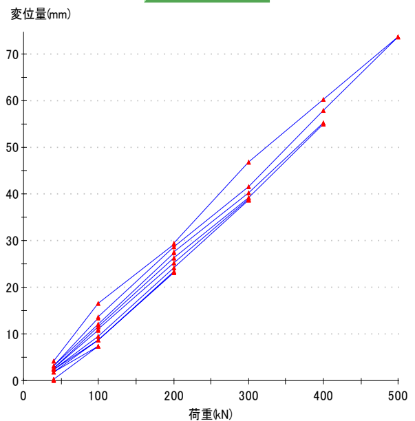
荷重-変位量曲線
