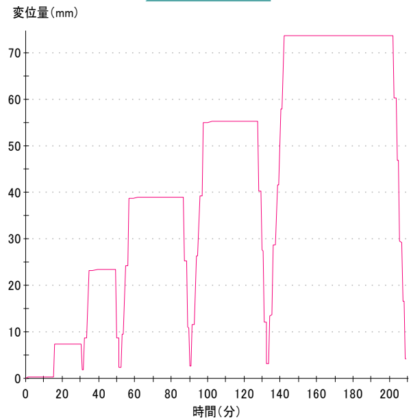
時間-変位量曲線
