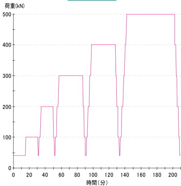
時間-荷重曲線
